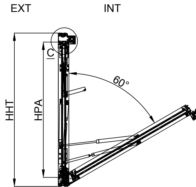
COUPE B-B
